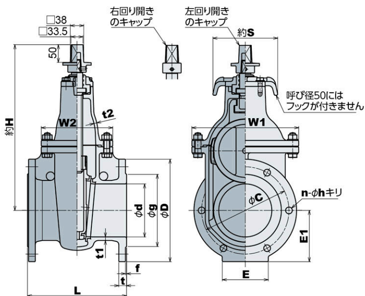
水道用ダクタイトル鋳鉄仕切弁 MM-C型(呼径50~300)
