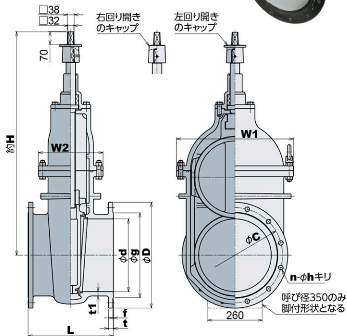
水道用ダクタイトル鋳鉄仕切弁 MMシール型(呼径350~500)
